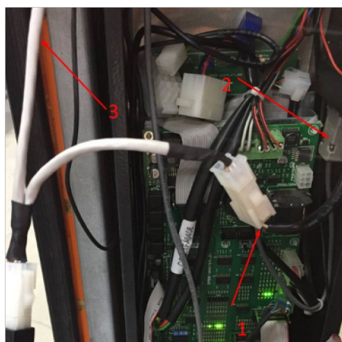
1. Подключение вилки MDBк плате автомата
