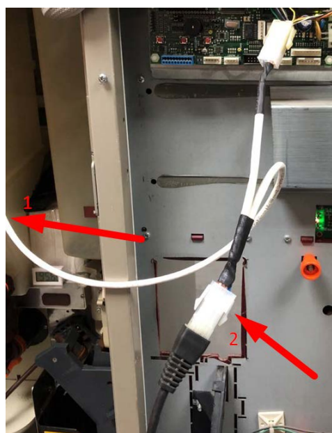
1.розетка AUX 2. Вилка MDB
