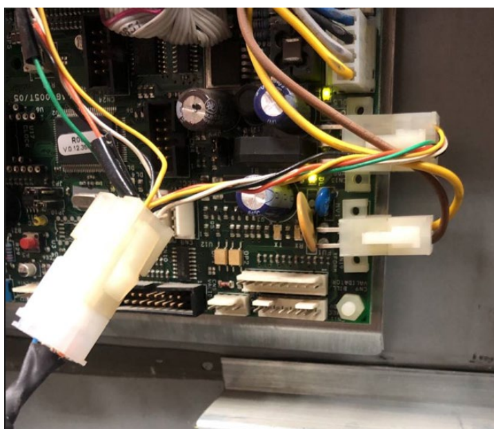
Подключение вилки MDB к плате автомата
